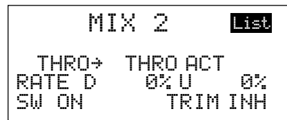
Mischer 2 (Seite 70)
